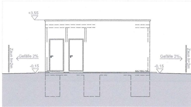
ANSICHT Ost
