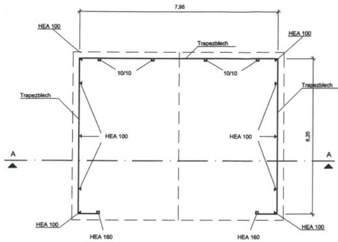
Grundriss Überdachung 1
