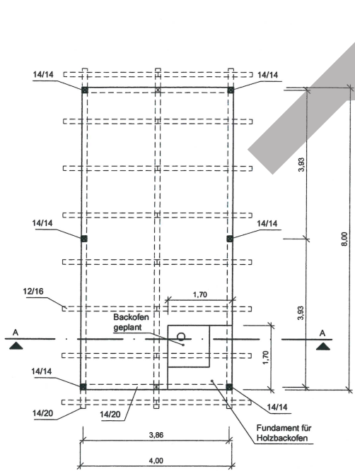
Grundriss
