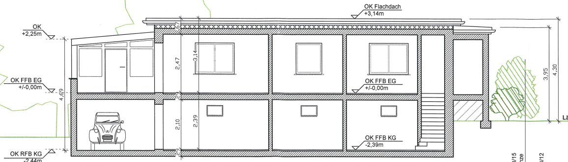
Längsschnitt L-L
