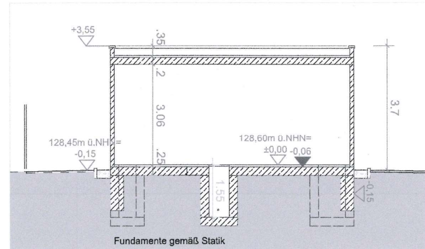
SCHNITT B-B
